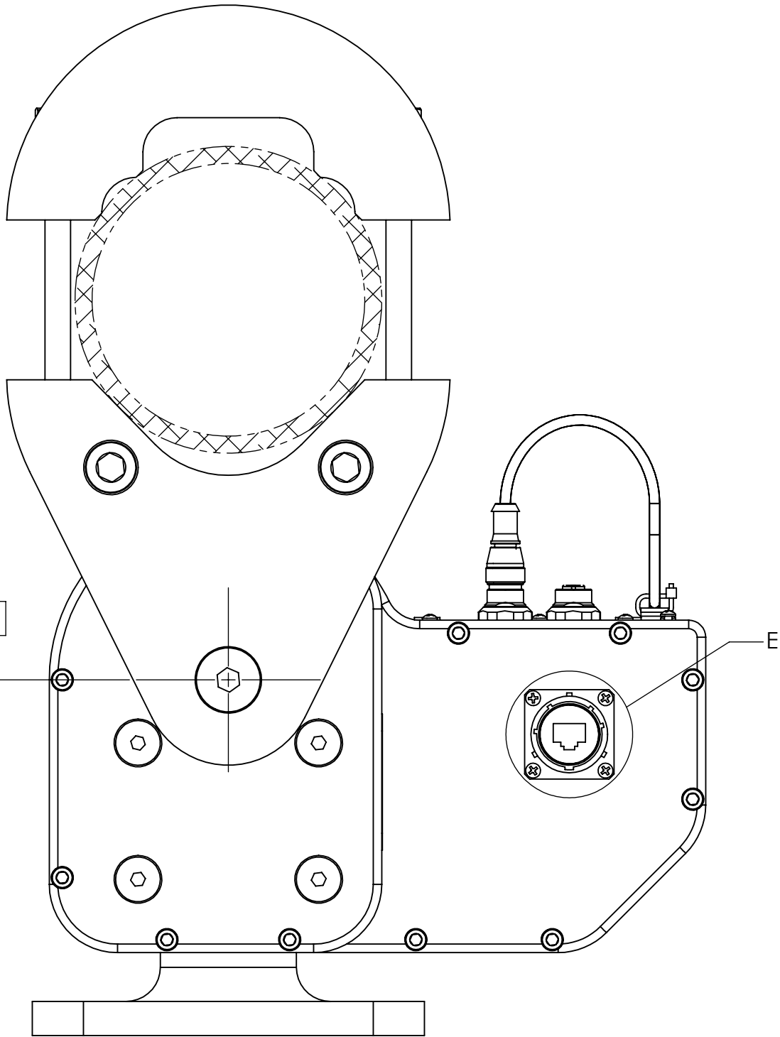
SECTION D-D
